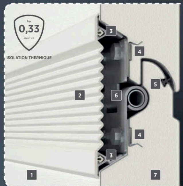
Porte PRIME, UniTherm
